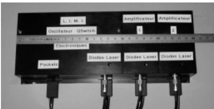
Photo 1 – LIMi, Laser Impulsionnel Modulaire Intégré
